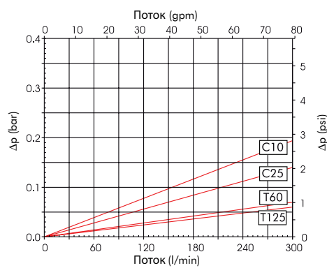
Перепускной клапан FA-2-10/11/20/21
