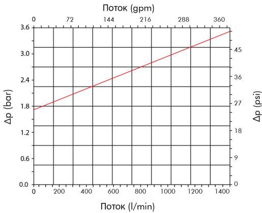
Перепускной клапан FCR-7- 30/31/32/33
