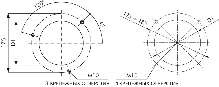
ДВА ВИДА РАСПОЛОЖЕНИЯ КООРДИНАТ КРЕПЕЖНЫХ ОТВЕРСТИЙ
