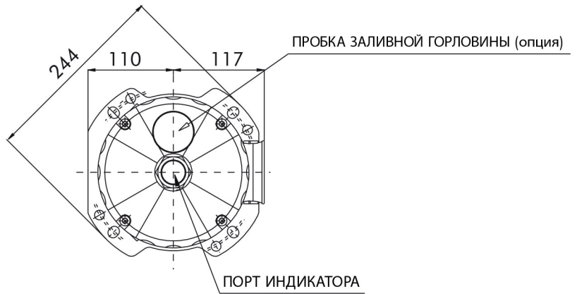
ДВА ВИДА РАСПОЛОЖЕНИЯ КООРДИНАТ КРЕПЕЖНЫХ ОТВЕРСТИЙ
