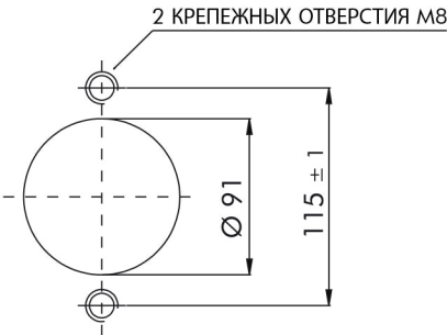
СХЕМА УСТАНОВКИ В БАК
