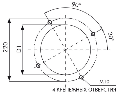
ДВА ВИДА РАСПОЛОЖЕНИЯ КООРДИНАТ КРЕПЕЖНЫХ ОТВЕРСТИЙ
