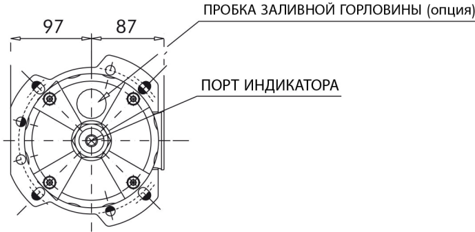
ДВА ВИДА РАСПОЛОЖЕНИЯ КООРДИНАТ КРЕПЕЖНЫХ ОТВЕРСТИЙ
