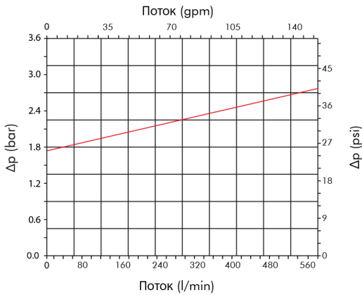
Перепускной клапан FCR-7- 20/21/22
